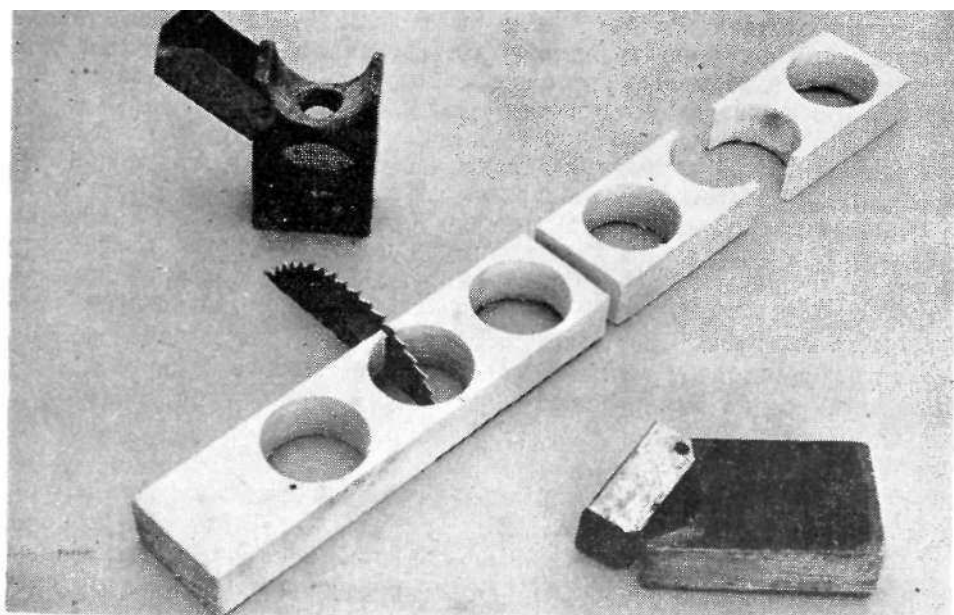
Рис. 137 — Клеточка Ванклера. Чтобы маточники, вырезанные из сота, можно было надежно защитить сверху, над углубленным отверстием, делают колпачок из тонкой жести
